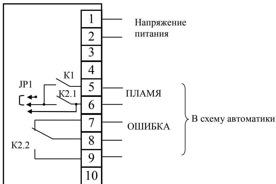
Рис. 4. Схема подключения датчика-реле пламени ПАРУС-002УФ-1/**Е.
